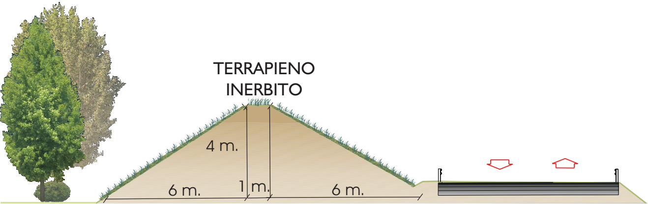
SCHERMATURA ARBOREA
