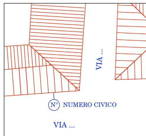
PROFILO STRADALE PIANTA DELLE COPERTURE SCALA 1:200
